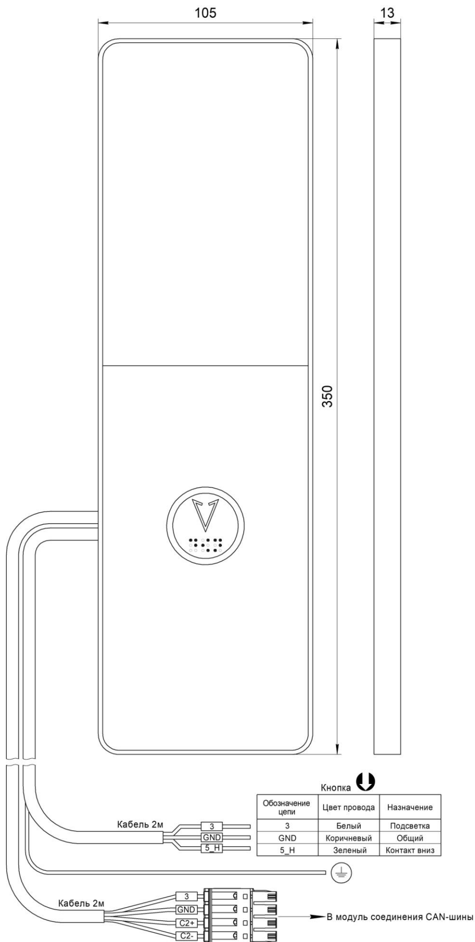
Рис.1 Внешний вид, габаритные и установочные размеры Вызывного поста МАЛАХИТ НШЕК.468381.015-01
